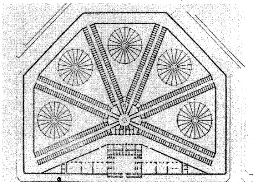
LÁMINA 23. Plano de la prisión de Mazas. Cf. p. 253.
